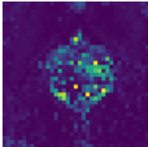
DINOv2-G-Reg4
