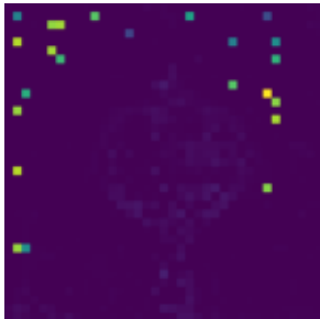
DINOv2-G
